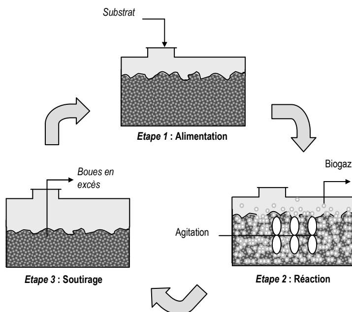
Figure 1 : Description des différentes étapes du cycle de fonctionnement d'un réacteur de méthanisation voie sèche
