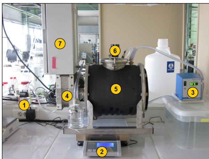
Figure 2 : Réacteur anaérobie « voie sèche » de laboratoire
